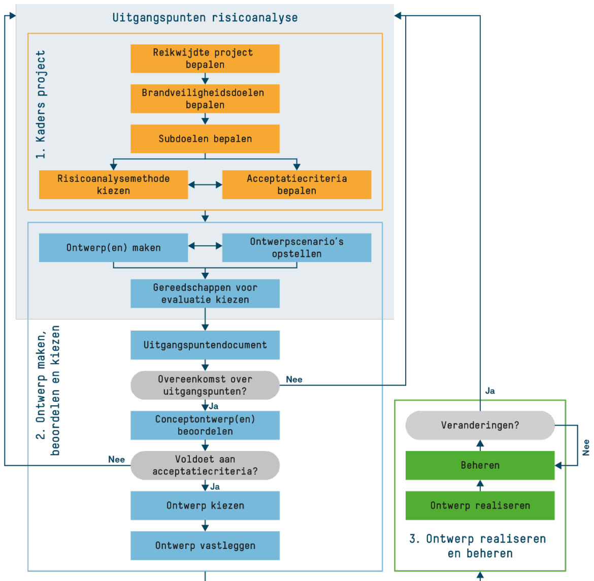
Figuur 3.4 Proces voor doelgerichte brandveiligheid voor gebouwen in Nederland
