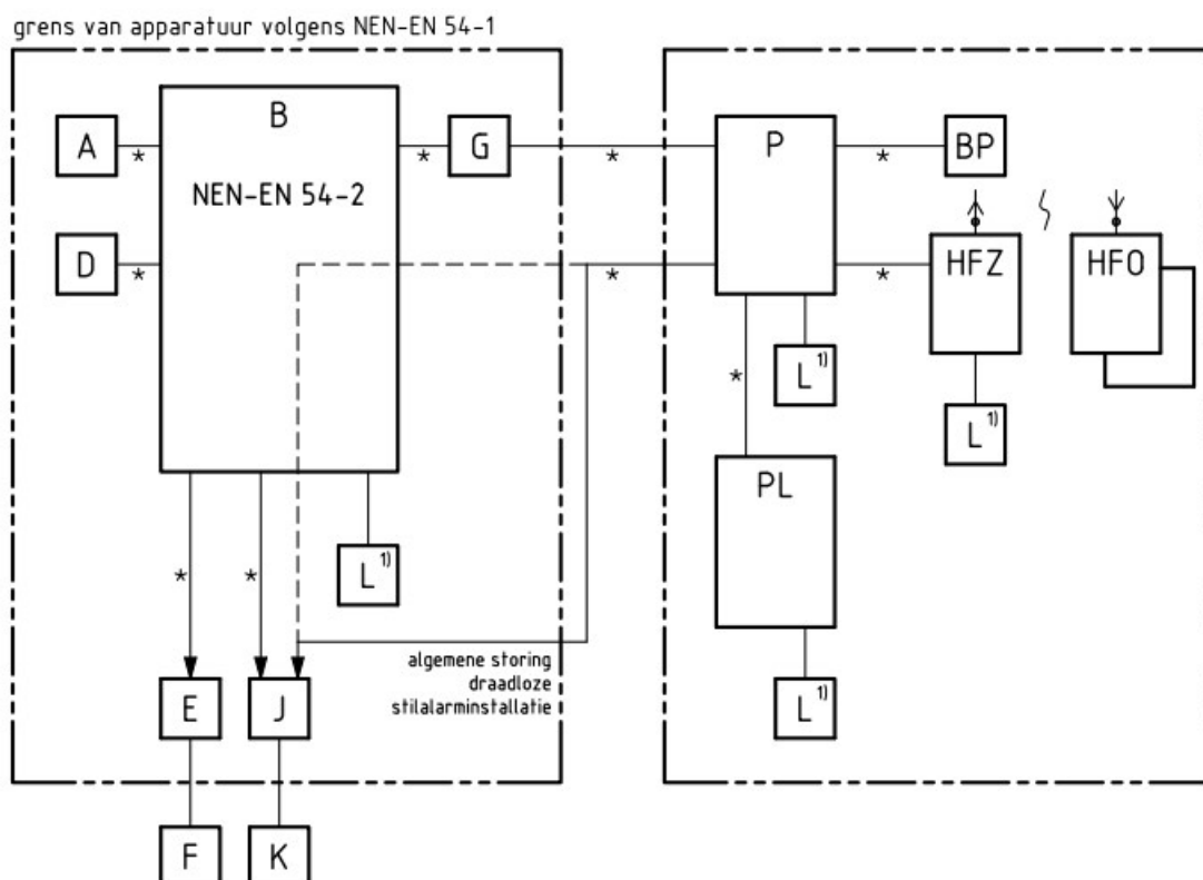
Legenda (lettercodering apparatuur is grotendeels overeenkomstig NEN-EN 54-1)
