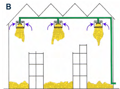
Figuur 8.9 (B) is een Hi-Ex inside airsysteem
