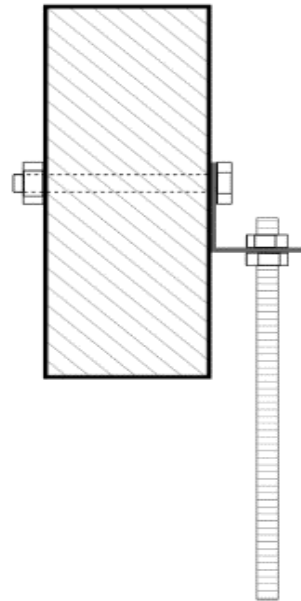
Figuur 11.1 Doorgaande bout-bevestiging door het verticale deel Bron: K. Boerma
